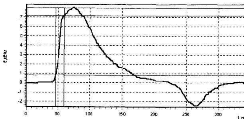
Рисунок П.3.2 - Пример осциллограммы напряженности электрической составляющей ИЭМП.
